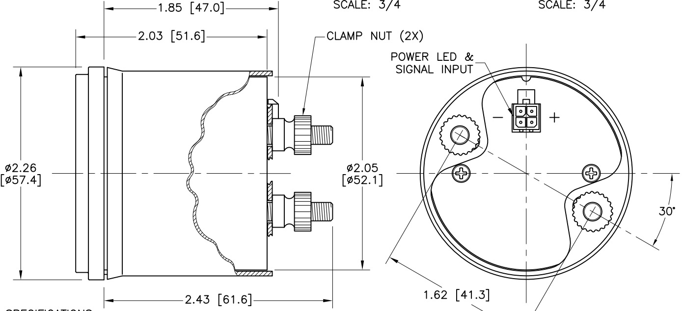
P/N 010-212-3W-1 SCALE: 3/4
