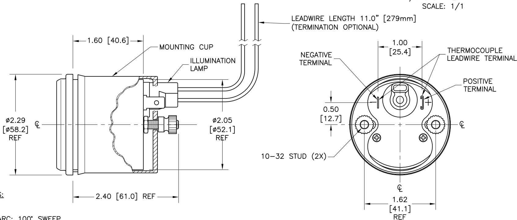
P/N 010-112-1R-1 SCALE: 1/1
