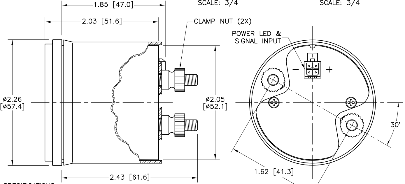
P/N 120-22W-3W-1 SCALE: 3/4
